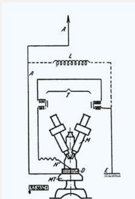
Schemat radiomikroskopu Czochralskiego
